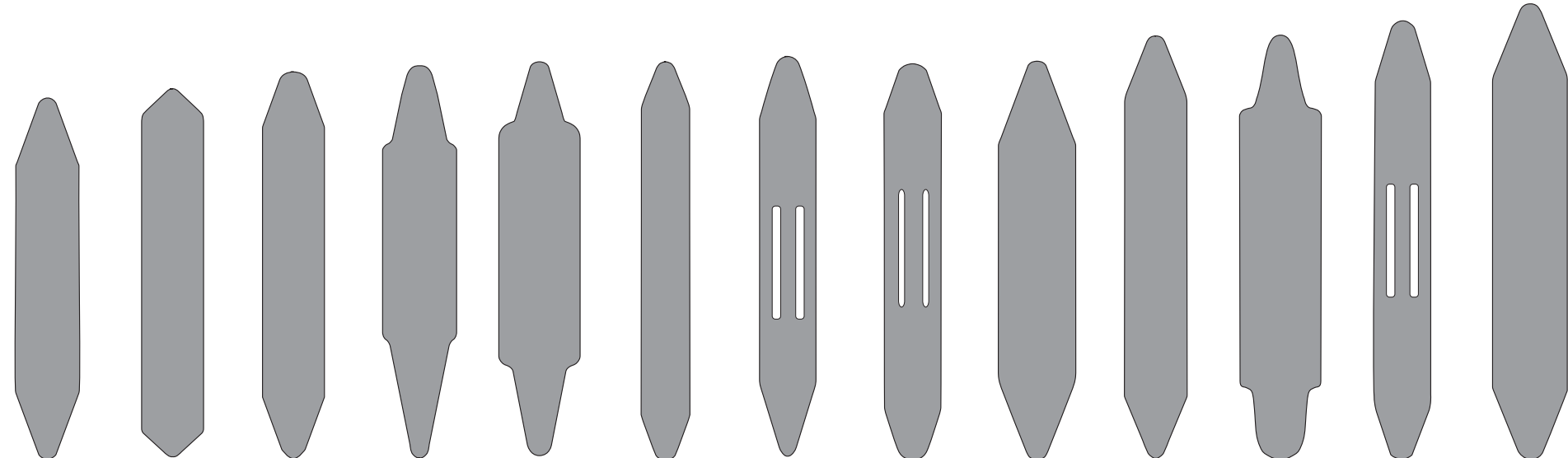
SP 5810 58 x 10 411 SP 5910 59 x 10 412 SP 6210 62 x 10 413 SP 6312 63 x 12 414 SP 63130 63 x 13 415 SP 6482 64 x 8 416 SS 649 64 x 9 417 SS 6490 63,5 x 9 418 SP 64125 64 x 12,5 424 SP 6810 68 x 10 419 SP 6813 68 x 13 420 SS 7090 70 x 9 421 SP 73120 73 x 12 425
