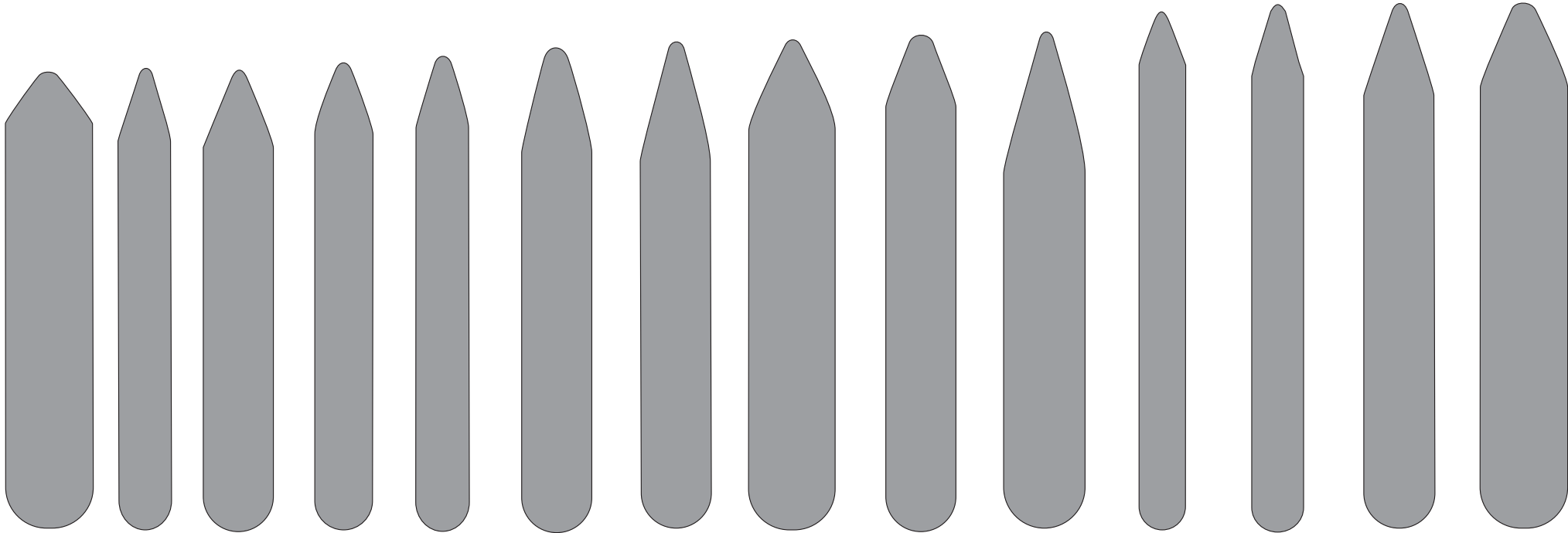
SP 7815 78 x 15 251 SP 799 79 x 9 253 SP 7912 79 x 12 252 SP 801 80 x 10 262 SP 829 82 x 9 254 SP 8312 83 x 12 275 SP 83120 83 x 12 282 SP 8415 84 x 15 279 SP 8512 85 x 12 255 SP 8514 85 x 14 256 SP 898 89 x 8 257 F-SP 909 90 x 9 322 SP 9012 90 x 12 266 SP 9015 90 x 15 258
