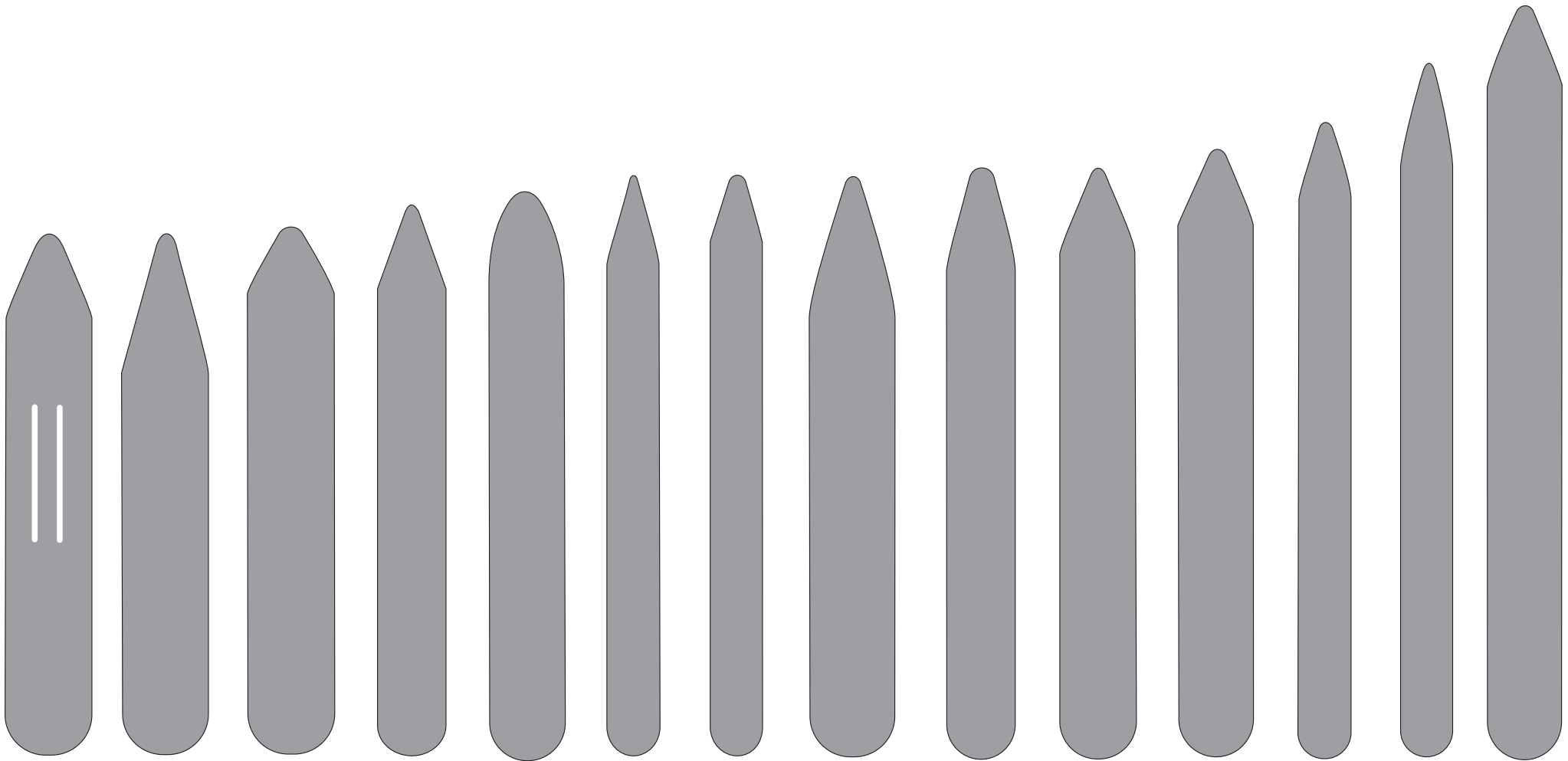
SP SP SP SP SP SP SP SP SP SP SP SP SP SP 9015 90150 9115 9512 9813 1009 10091 10015 10212 10213 10513 1109 1209 13013 90 x 15 90 x 15 91 x 15 95 x 12 98 x 13 100 x 9 100 x 9 100 x 15 102 x 12 102 x 13 105 x 13 110 x 9 120 x 9 130 x 13 265 273 283 319 264 259 271 280 281 261 272 260 274 269
